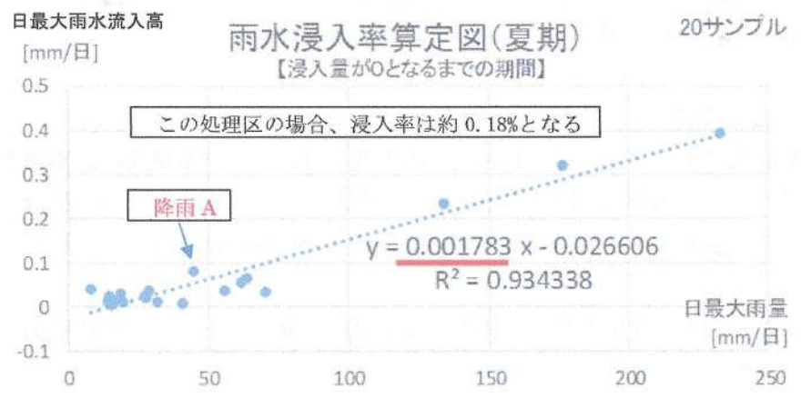
図 3-3 雨水流入高と雨量の相関図の例（日最大）
