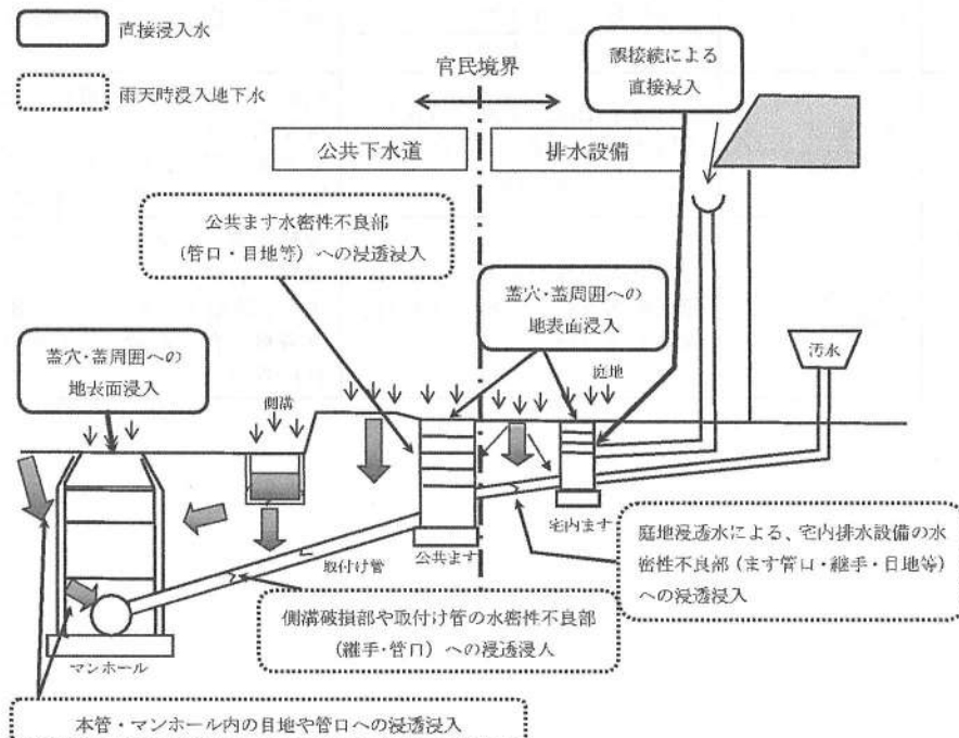
図 3-1 雨天時浸入水の浸入経路のイメージ
